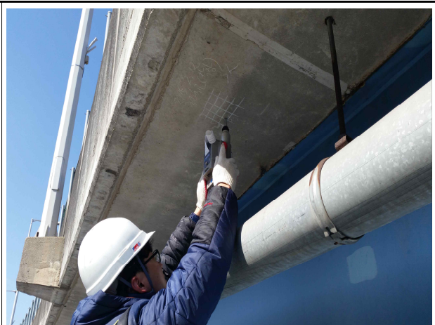
반발경도시험
